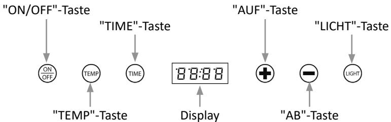
Bedienelemente
