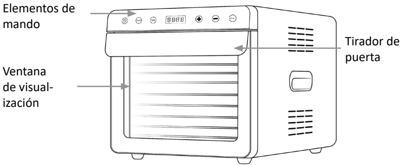
Lado delantero
